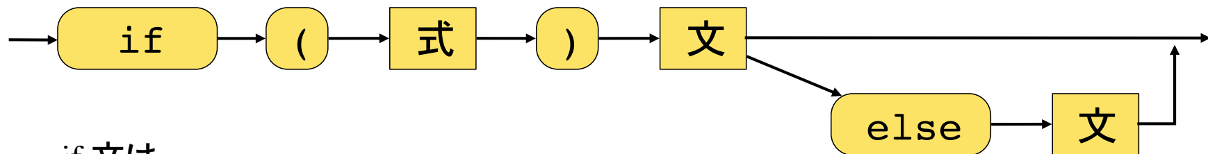
if 文の構文図
