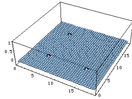
迷路模様
