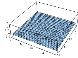
リング波
